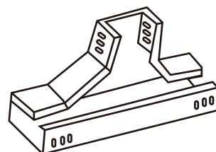
下边垂直三通
