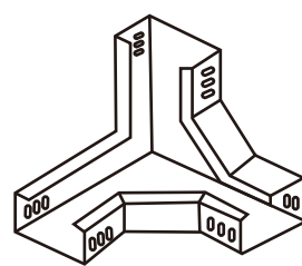
下角垂直三通
