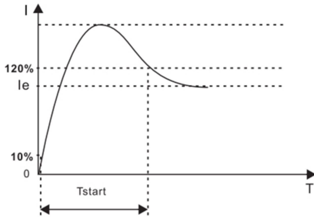
I:运行电流； Ie:额定电流，由用户自行整定； Tstart:电动机启动时间。
