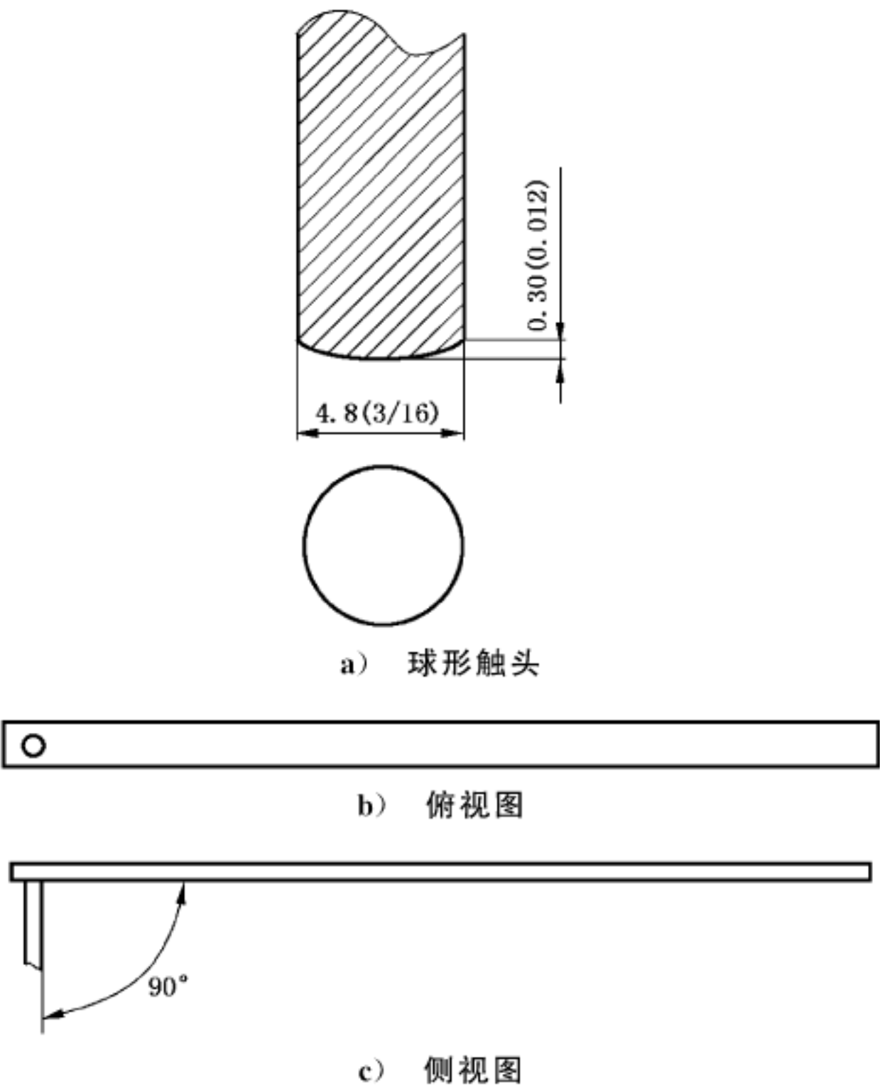
图 D.25 典型的 90°钩形工具示例
