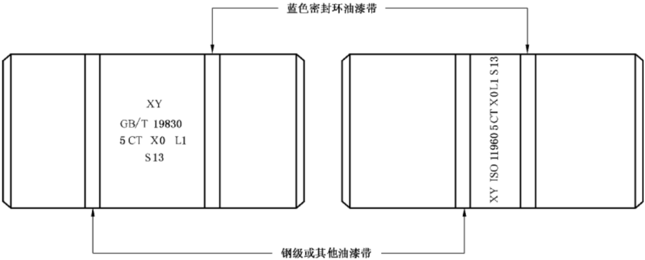
图 D.29 密封环油漆带示例
