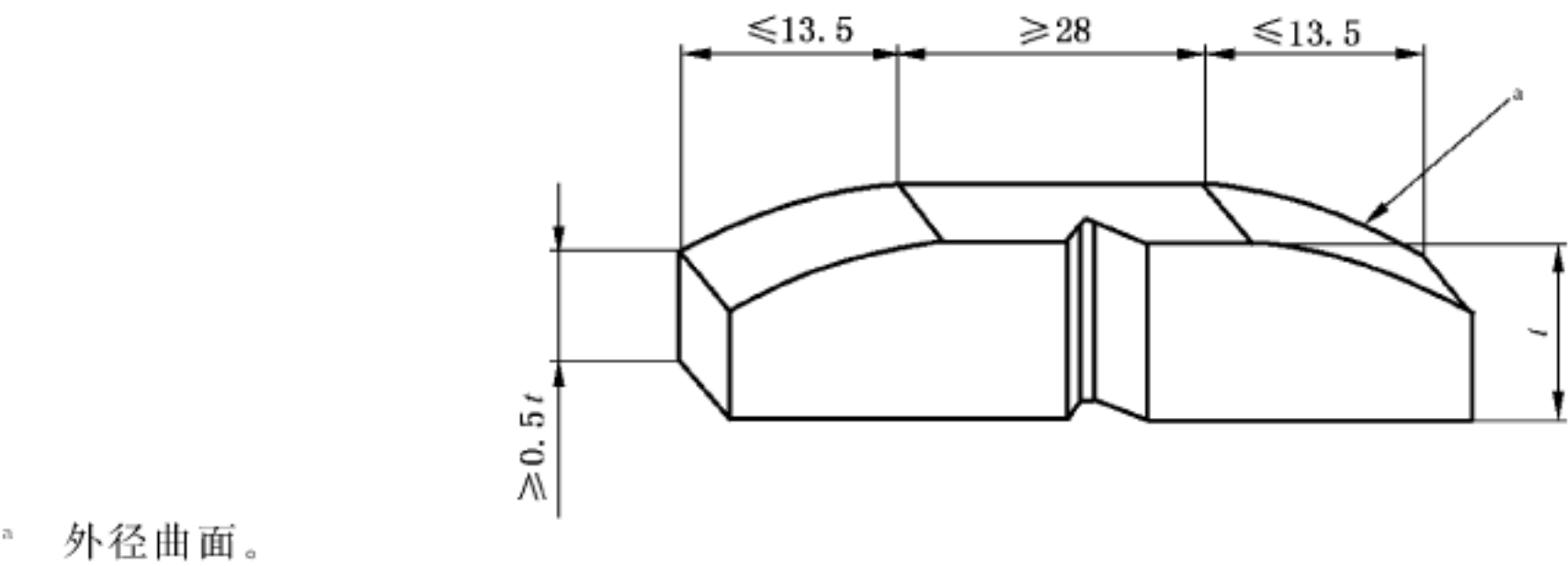
图 D.21 SR16.1 允许保留外径曲面的试样要求
